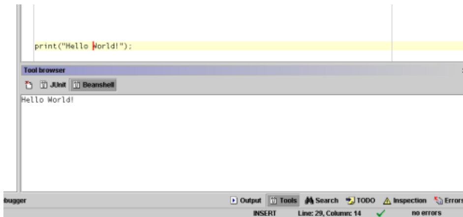
Interpreteur Beanshell
